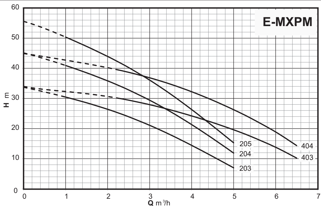
Kennlinien n \approx 2900 1/min
