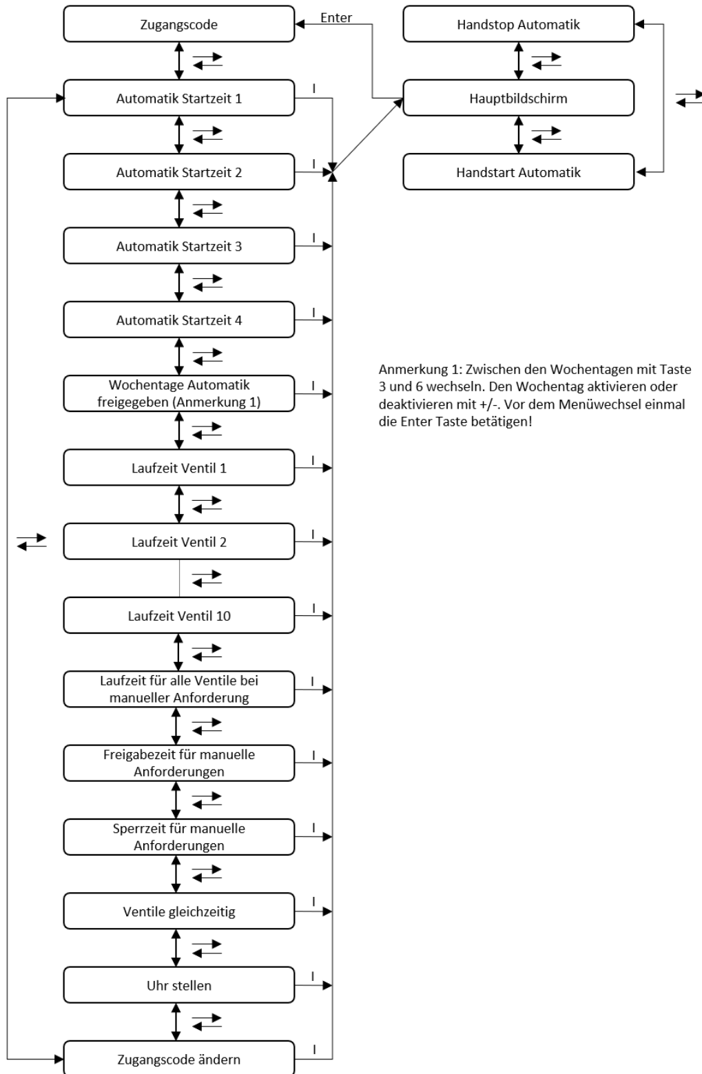
Abbildung 4.2.1: Menüstruktur
