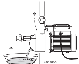
Fig. 5 Scarico Draining Entleerung Vidange Vaciado Avtapping Aftappen Αποστράγγιστο Слив 排空
